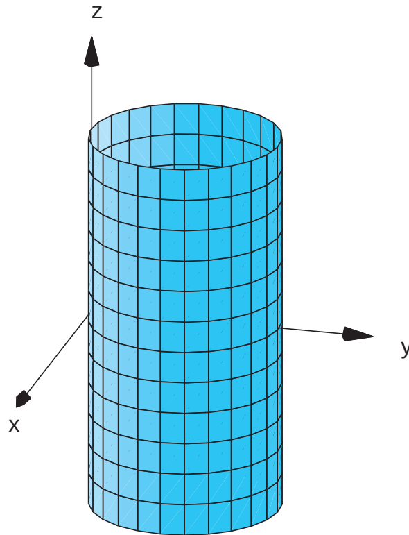
Figura 6.46: Cilindro circular de equação em coordenadas cilíndricas r = a \sin \theta
