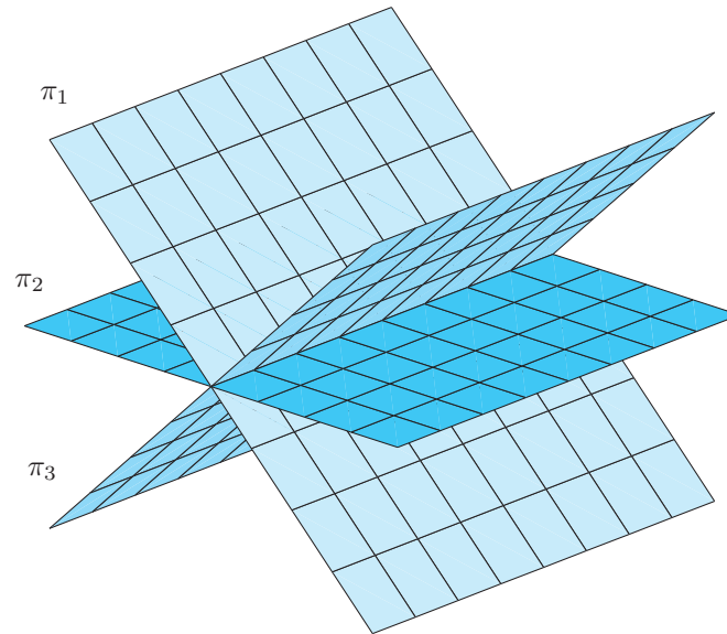
Figura 4.41: Reta interseção de 3 planos
