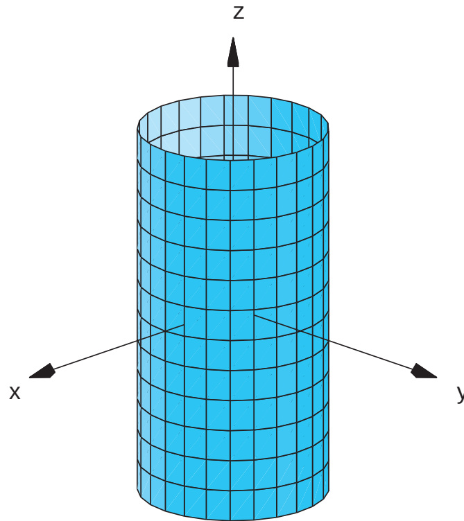
Figura 6.50: Cilindro circular de equação em coordenadas esféricas r \sin \phi = a
