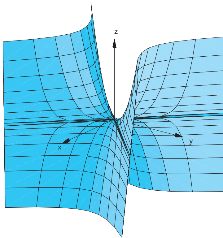
Figura 6.49: Parabolóide hiperbólico de equação em coordenadas esféricas r \sin^2 \phi \cos 2\theta = a^2 \cos \phi
