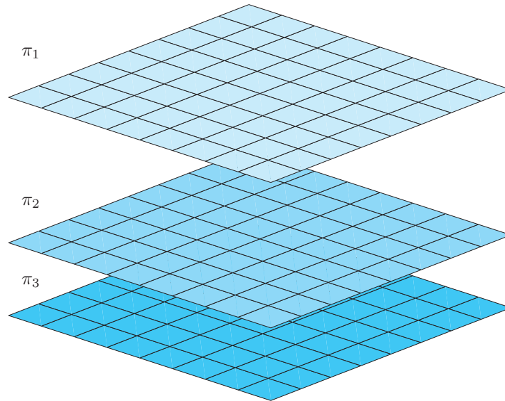
Figura 4.38: Três planos paralelos
