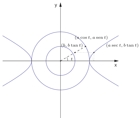
Figura 5.42: Hipérbole parametrizada usando secante e tangente
