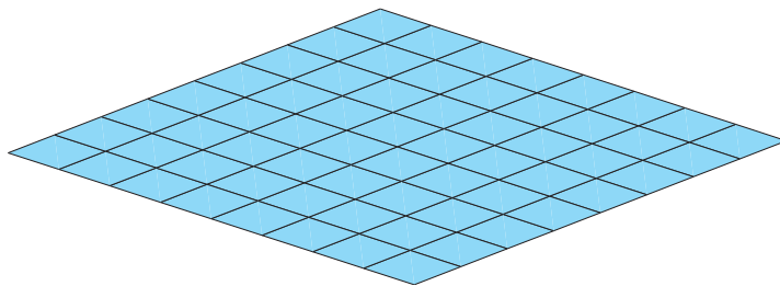
Figura 4.34: Dois planos paralelos
