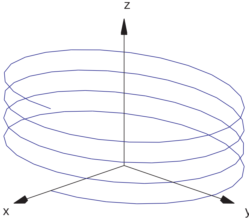
Figura 6.55: Hélice
