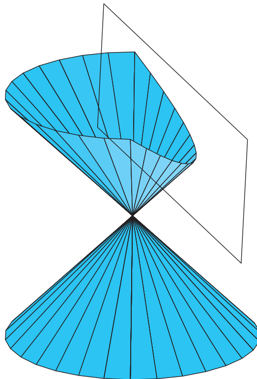
Figura 5.14: Parábola obtida seccionando-se um cone com um plano
