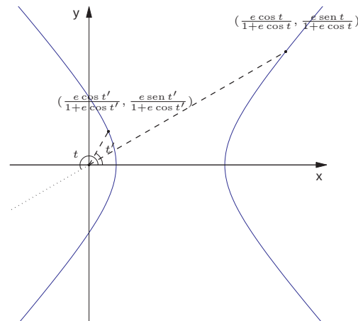
Figura 5.45: Hipérbole com foco na origem parametrizada usando a sua fórmula em coordenadas polares
