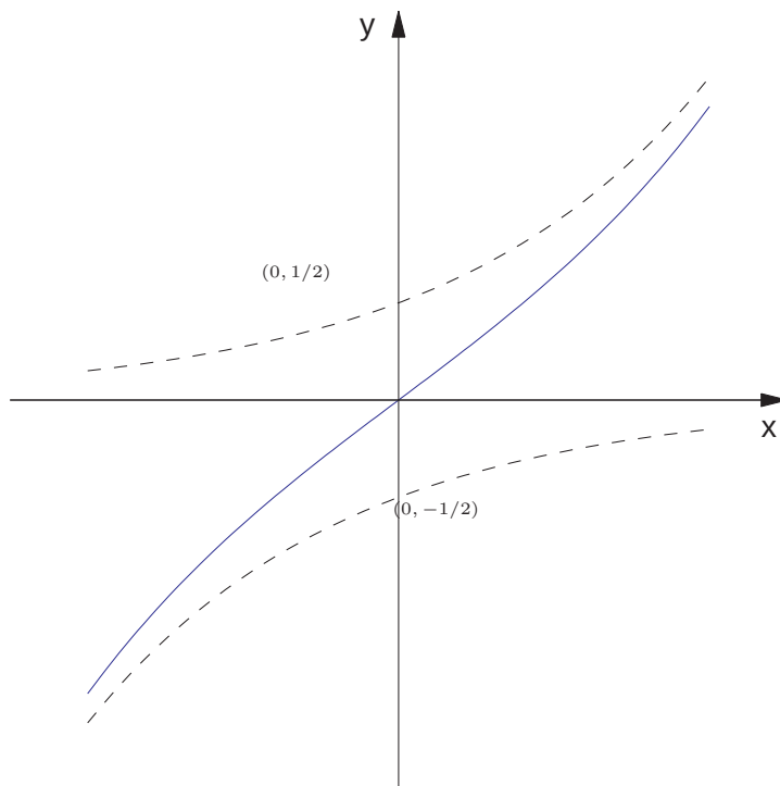
Figura 5.41: Seno hiperbólico
