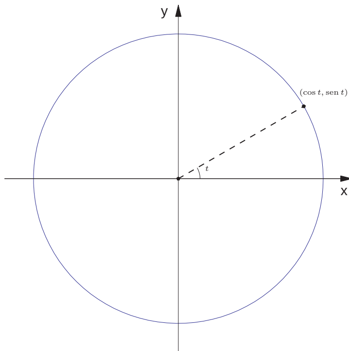
Figura 5.38: Circunferência parametrizada
