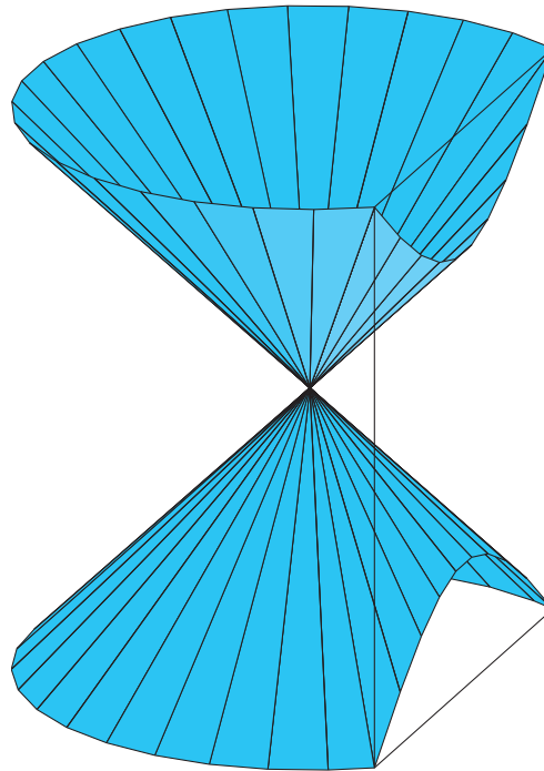
Figura 5.8: Hipérbole obtida seccionando-se um cone com um plano
