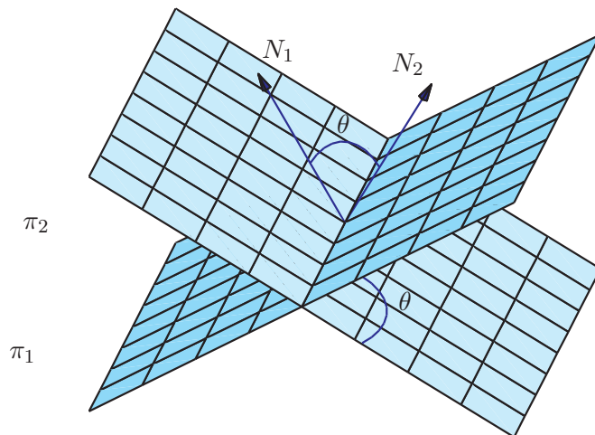
Figura 4.25: Ângulo entre dois planos
