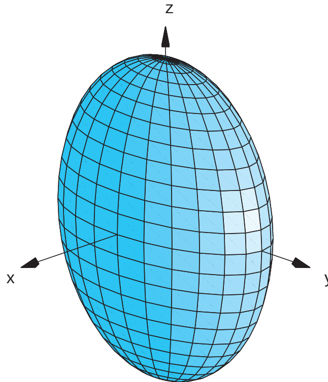
Figura 6.52: Elipsóide
