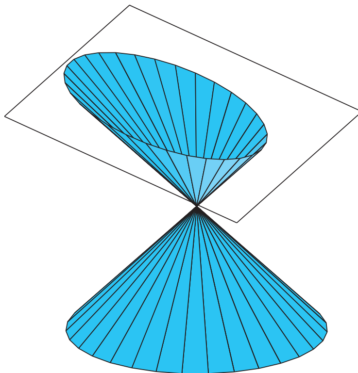
Figura 5.4: Elipse obtida seccionando-se um cone com um plano
