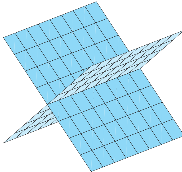
Figura 4.33: Dois planos que se interceptam segundo uma reta
