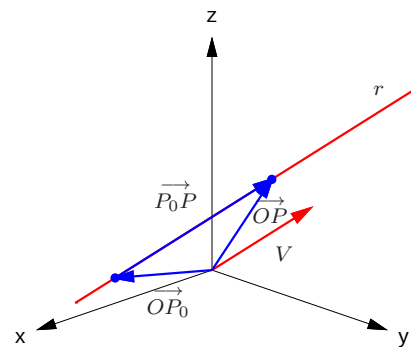
Figura 4.9: Reta paralela ao vetor V = (a, b, c)
