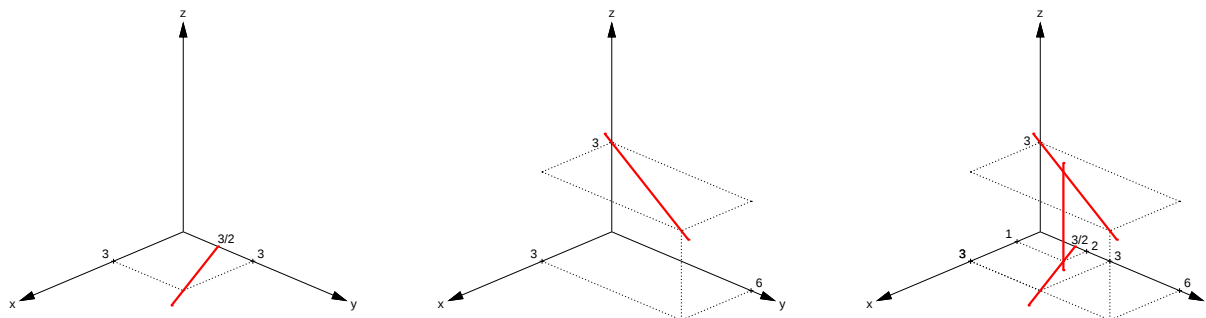
Figura 4.23: Retas r_1 , r_2 e r_3 do Exemplo 4.8
