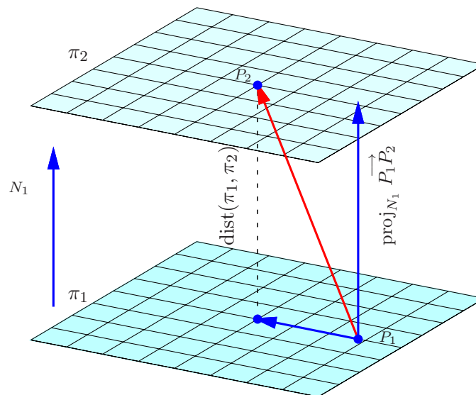
Figura 4.28: Distância entre dois planos
