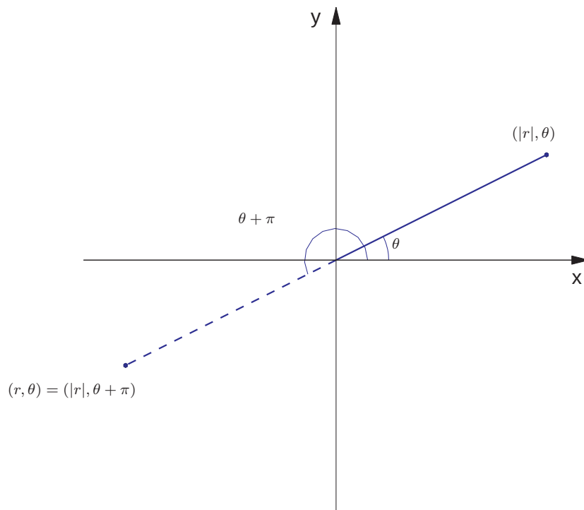
Figura 5.23: Para r < 0 , (r, \theta) = (|r|, \theta + \pi)
