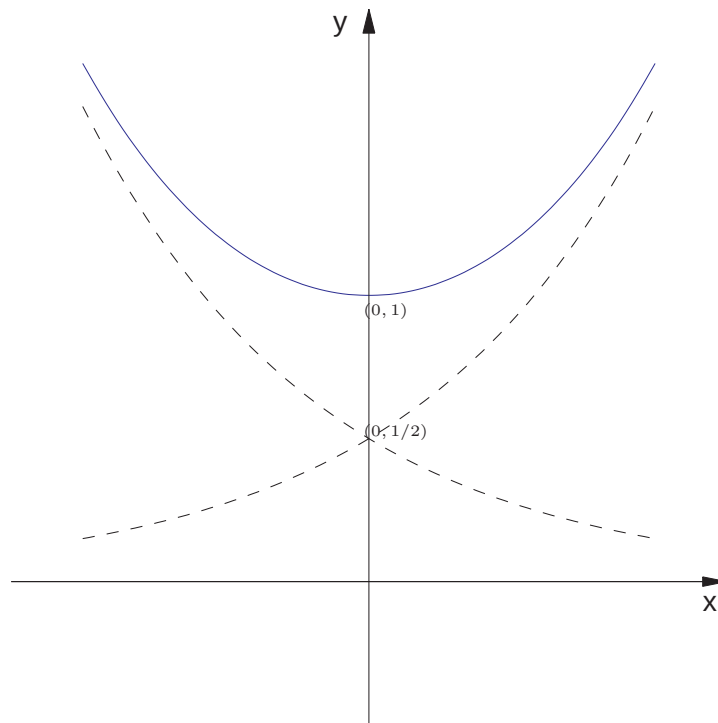
Figura 5.40: Cosseno hiperbólico
