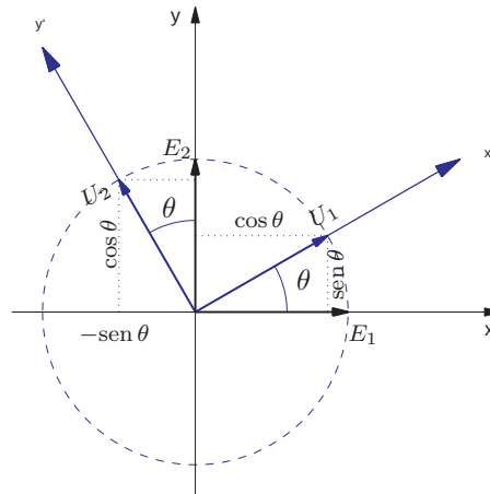
Figura 7.4: Rotação de um ângulo \theta
