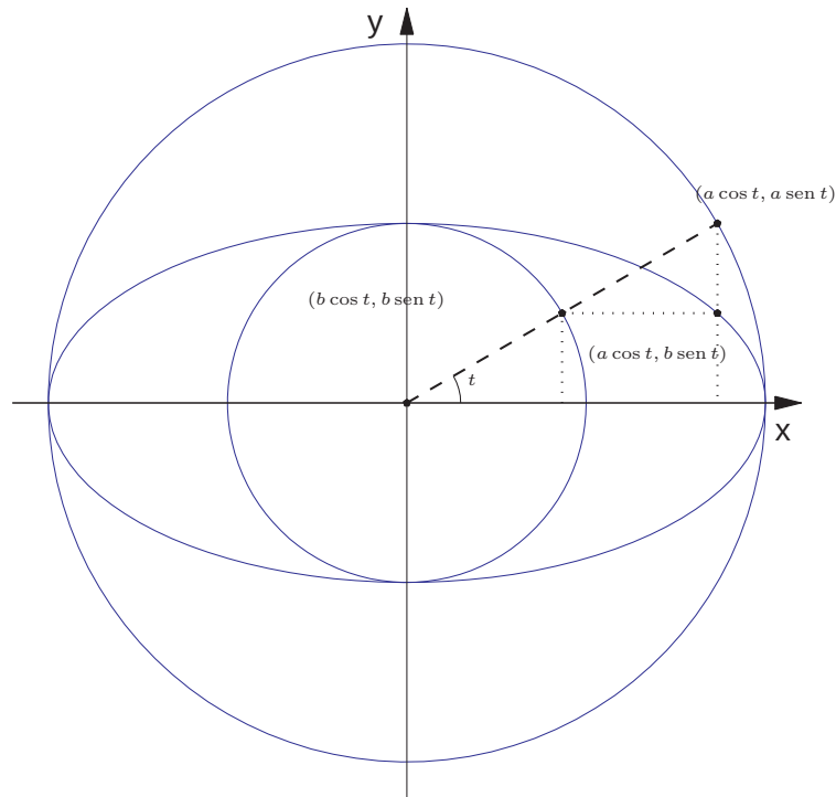
Figura 5.39: Elipse parametrizada
