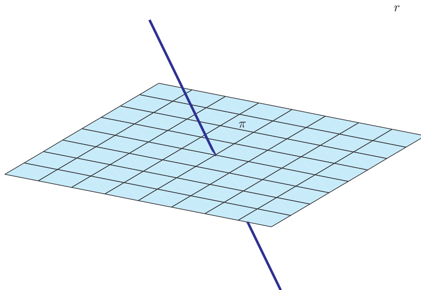
Figura 4.35: Reta e plano concorrentes
