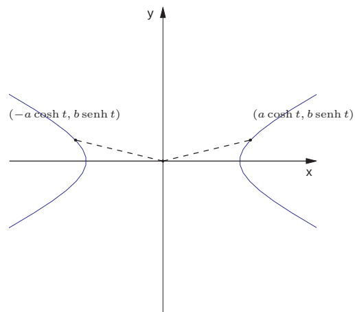
Figura 5.43: Hipérbole parametrizada usando as funções hiperbólicas
