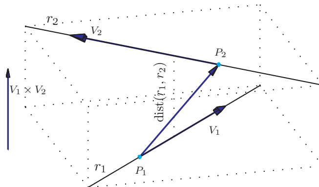
Figura 4.30: Distância entre duas retas reversas
