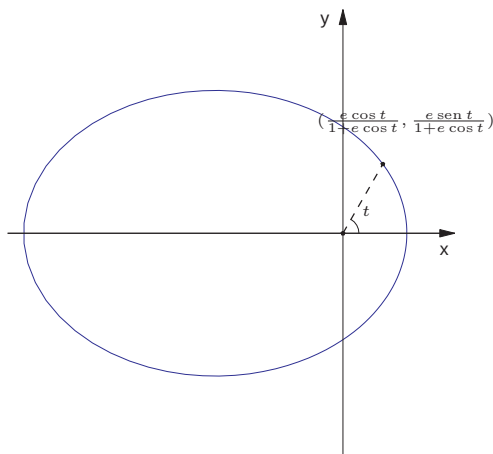
Figura 5.44: Elipse com foco na origem parametrizada usando a sua fórmula em coordenadas polares
