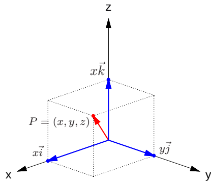
Figura 7.1: \vec{OP} = x\vec{i} + y\vec{j} + z\vec{k}
