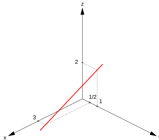
Figura 4.18: Reta que passa pelo ponto P_0 = (-3, 3/2, 4) paralela ao vetor V = (-6, 1, 4)
