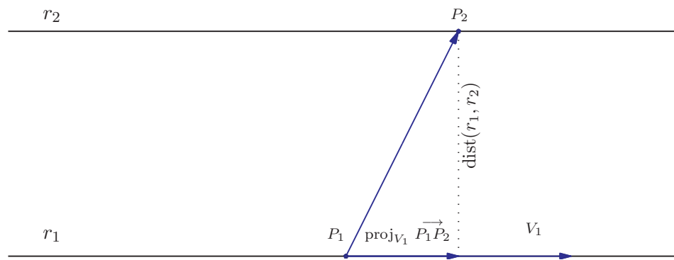
Figura 4.29: Distância entre duas retas paralelas
