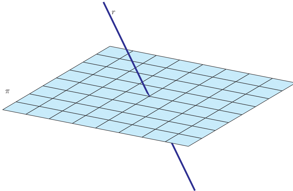
Figura 4.31: Reta e plano concorrentes
