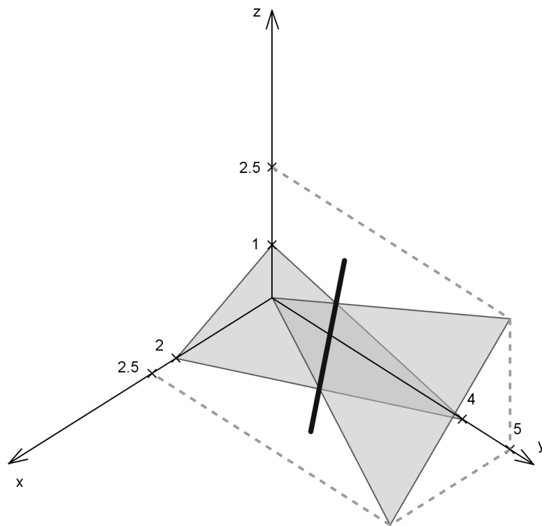
Figura 4.22: \pi_1 , \pi_2 e \pi_1 \cap \pi_2
