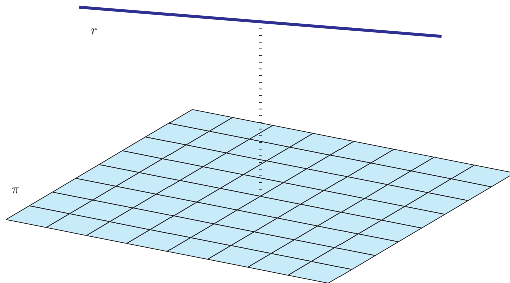
Figura 4.32: Reta e plano paralelos
