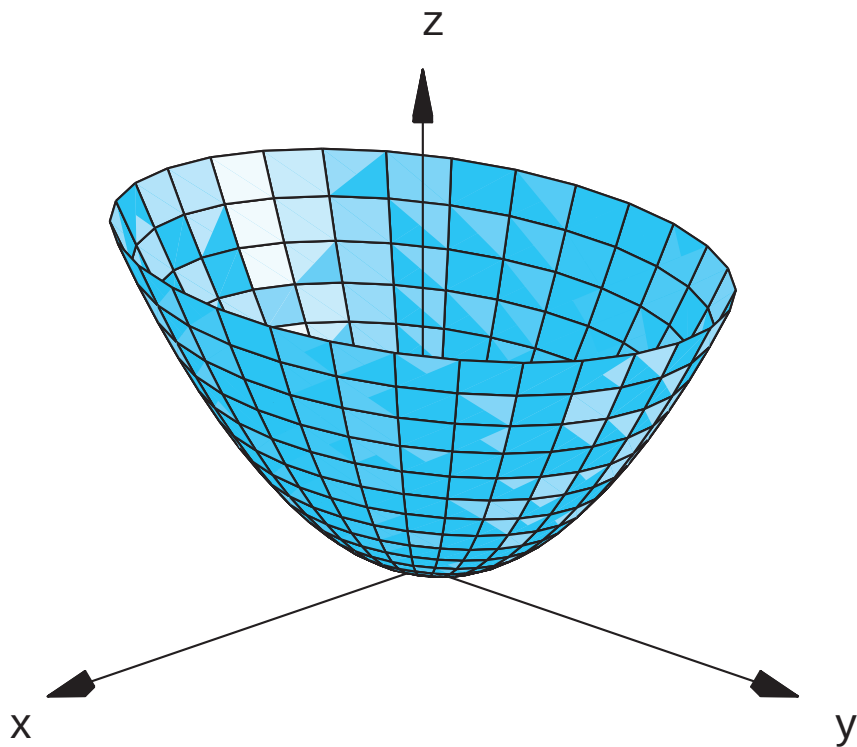
Figura 6.54: Parabolóide elíptico
