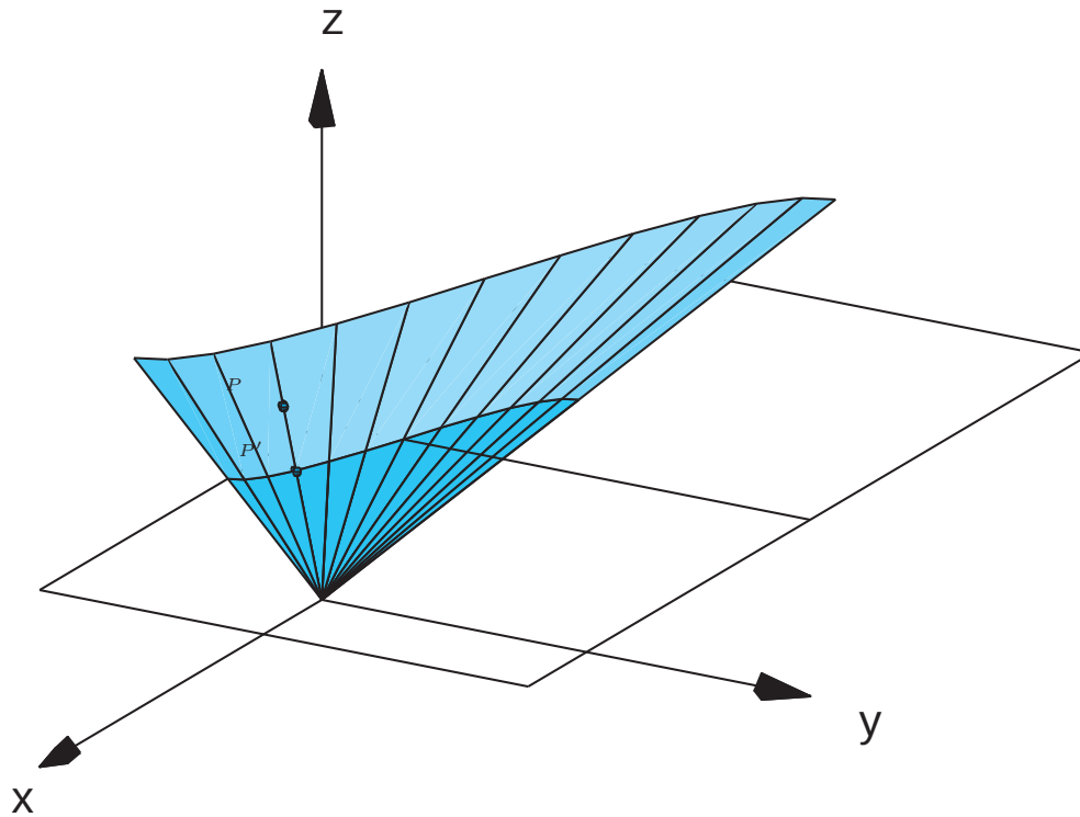
Figura 6.33: Superfície cônica
