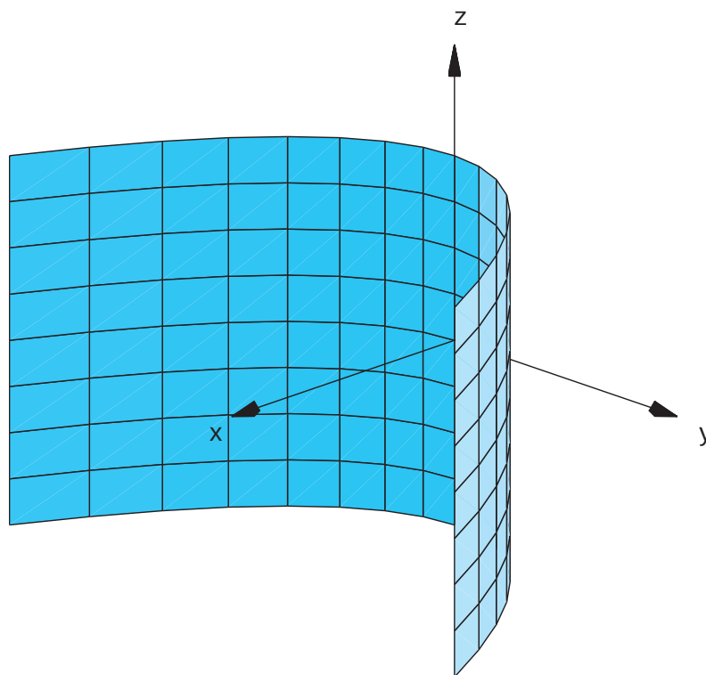
Figura 6.28: Cilindro parabólico de equação y^2 = 4px , p > 0
