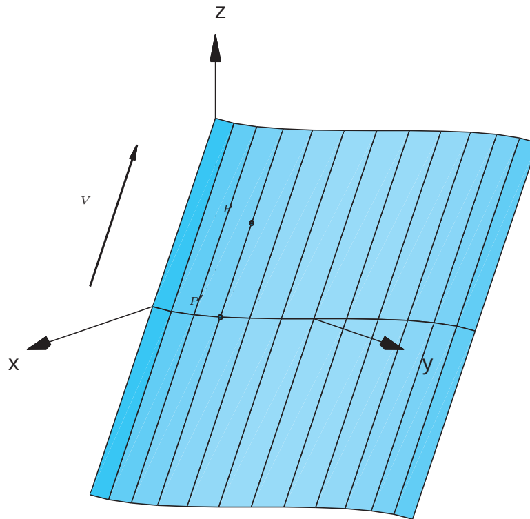
Figura 6.30: Superfície cilíndrica
