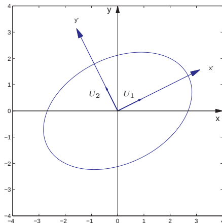
Figura 7.6: Elipse do Exemplo 7.4
