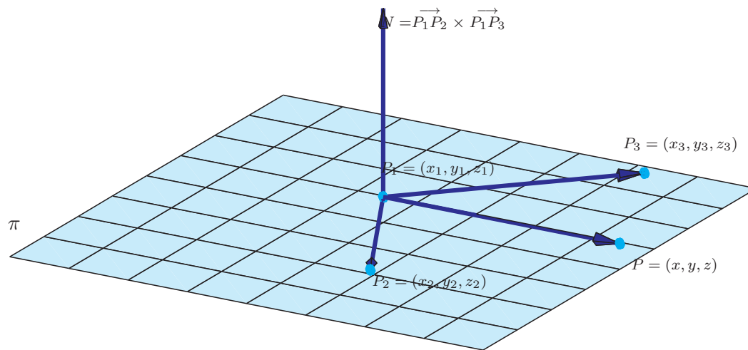
Figura 4.7: Plano que passa por três pontos
