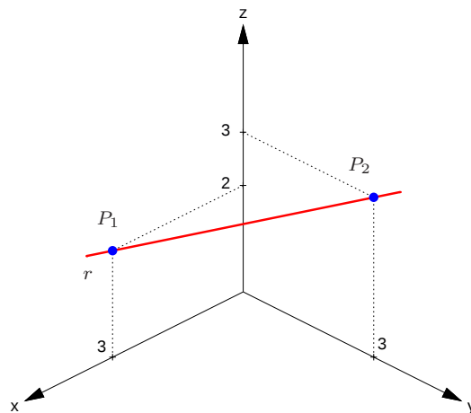
Figura 4.19: Reta que passa pelos pontos P_1 = (3, 0, 2) e P_2 = (0, 3, 3)
