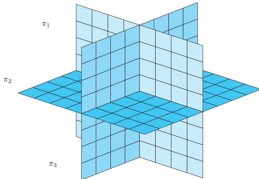
Figura 4.37: Três planos que se interceptam segundo um ponto
