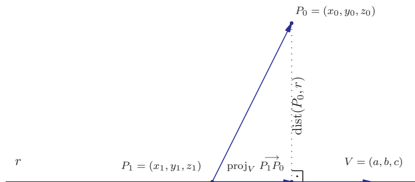
Figura 4.27: Distância de um ponto P_0 = (x_0, y_0, z_0) a uma reta r
