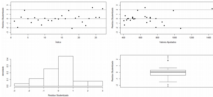
Figura 4: Análise residual para o modelo 2
