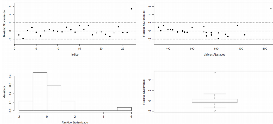
Figura 2: Análise residual para o modelo 1
