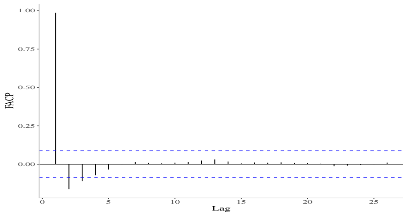
Figura: FACP da série simulada para um modelo ARIMA(1,1,1) com \phi = 0,8 e \theta = 0,8 .
