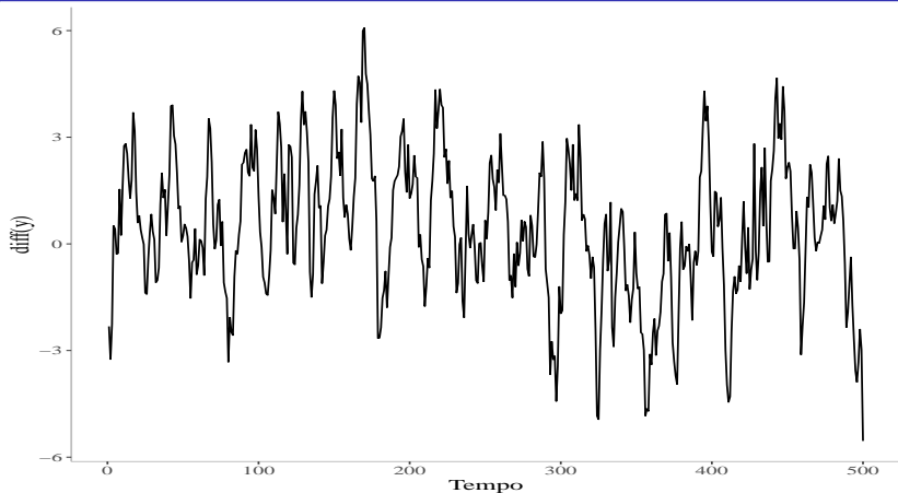
Figura: Primeira diferenças da série simulada para um modelo ARIMA(1,1,0) com \phi = 0,9 .
