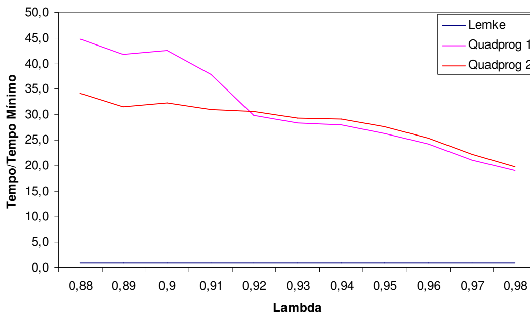
Figura 5.13 – Comparação das estratégias de resolução do subproblema (2.1) para a instância S&P.
